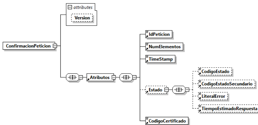
Figura 12. Mensaje ConfirmacionPetition
