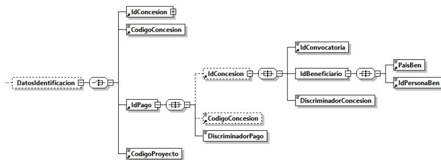
Figura 9. Respuesta - IdPago
