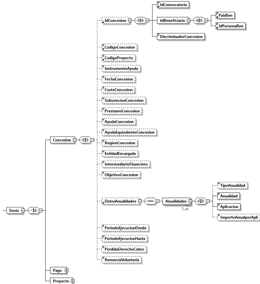
Figura 3. Petición - Concesion
