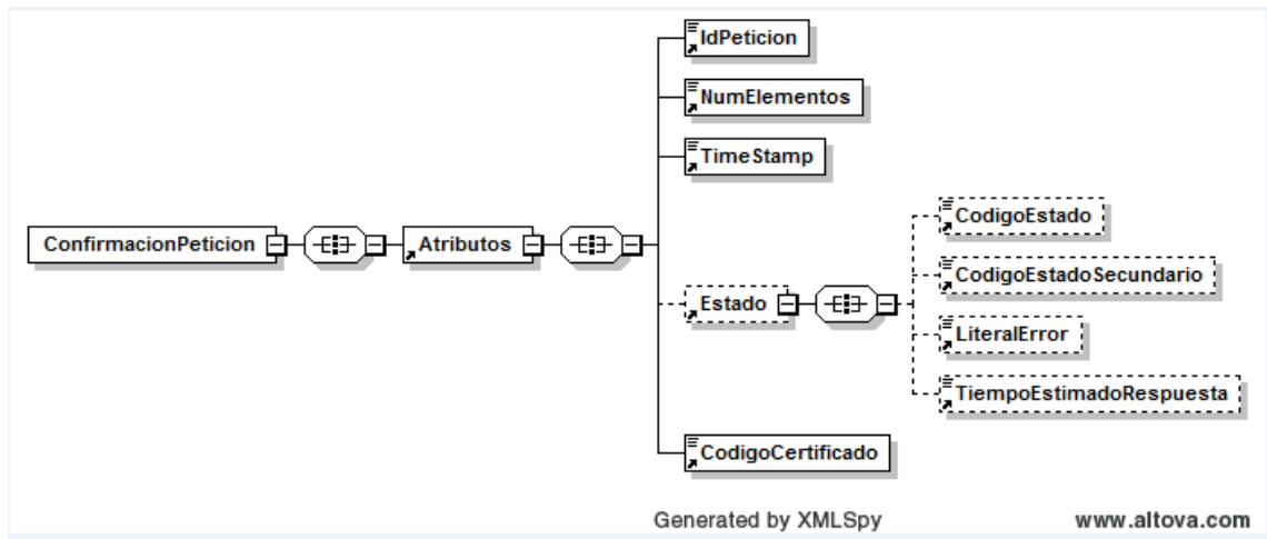
Figura 5.- Mensaje ConfirmacionPeticon
