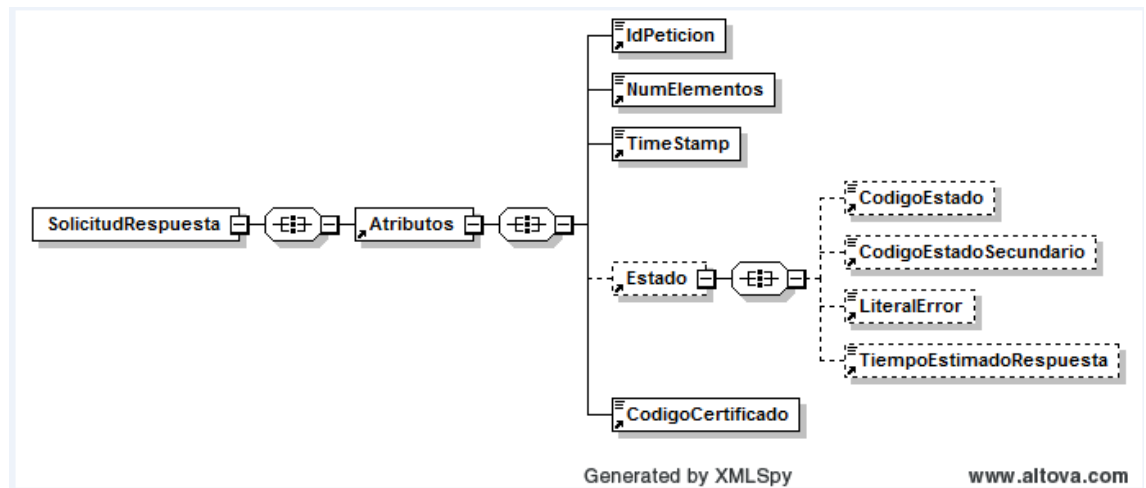
Figura 6.- Mensaje SolicitudRespuesta
