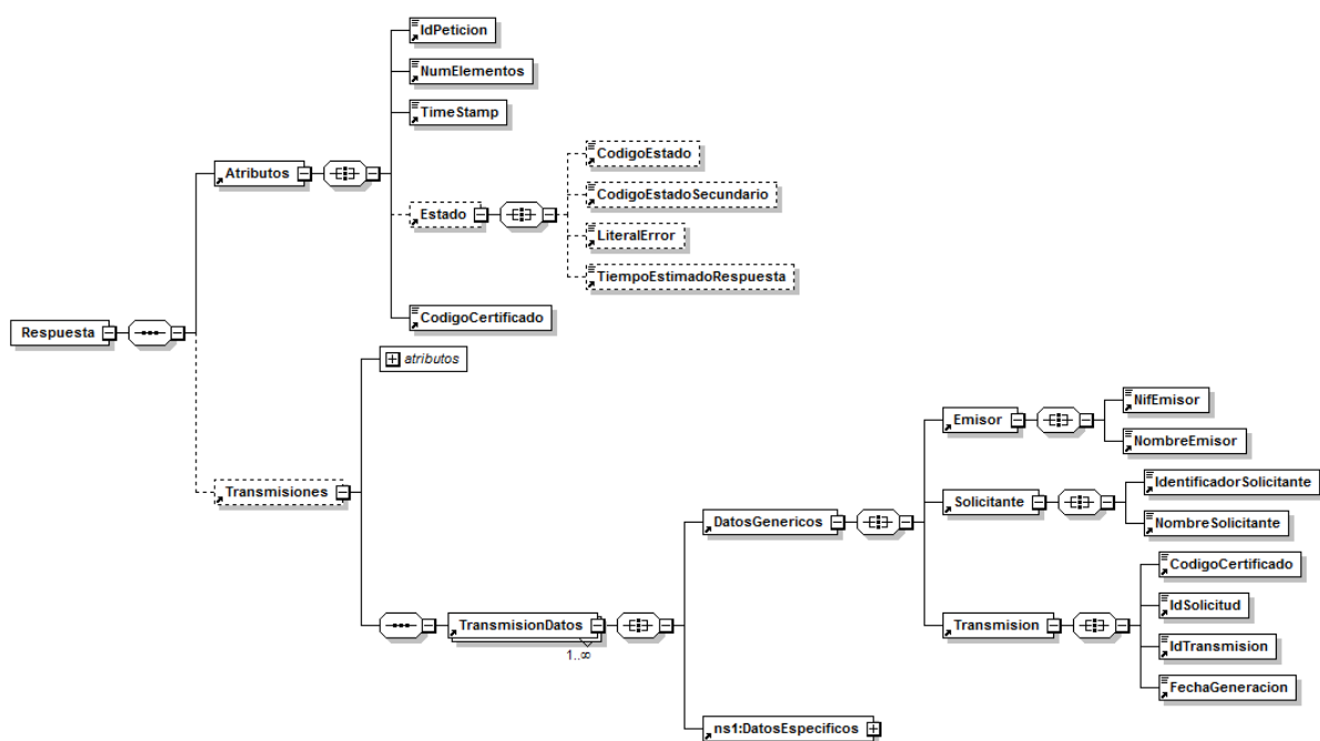
Figura 3.-Respuesta SCSPv3
