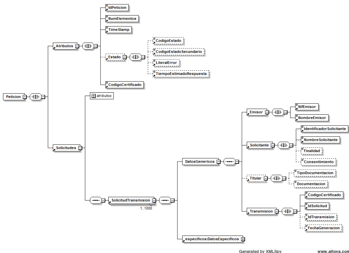
Figura 1.- Petición
