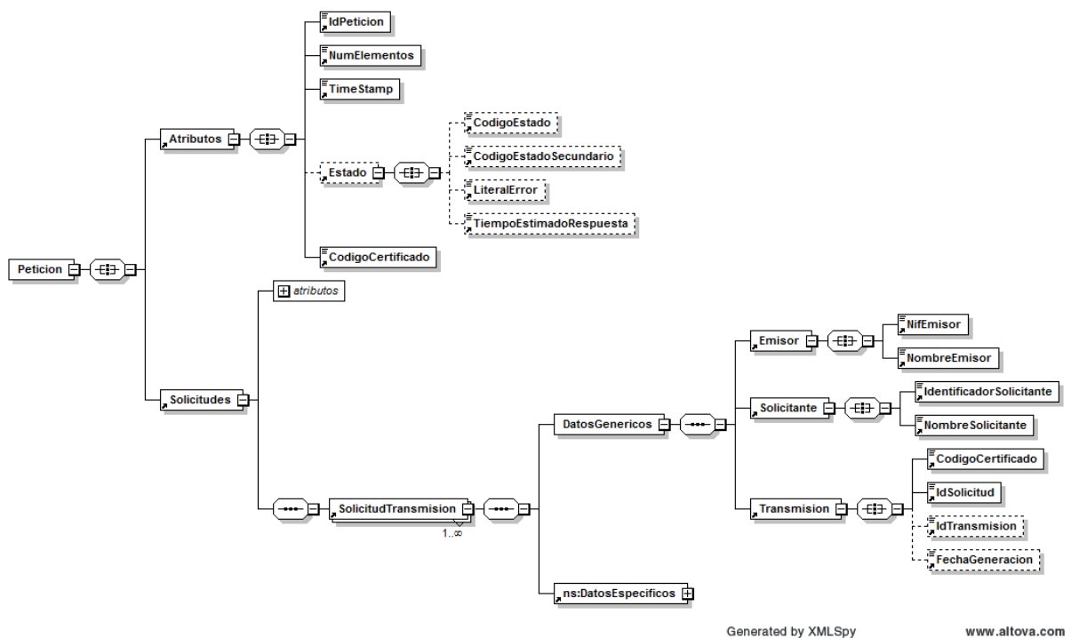
Figura 1.- Petición
