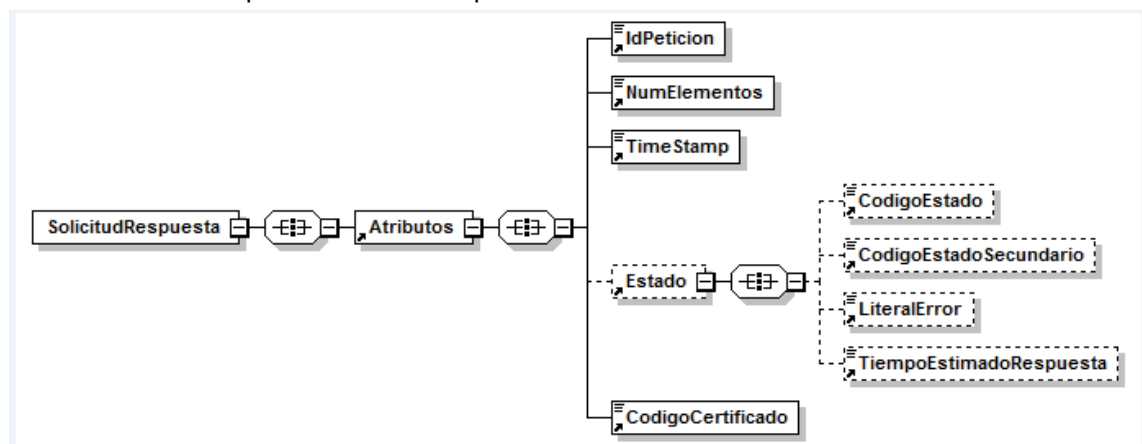
Figura 6.- Mensaje SolicitudRespuesta
