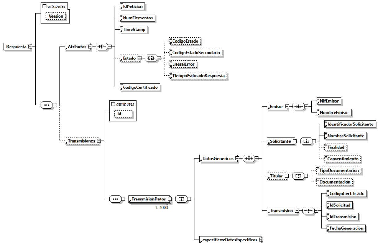
Figura 5. Mensaje Respuesta
